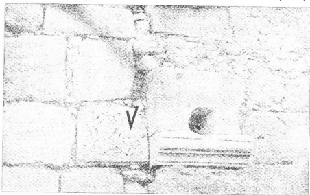
Рис. 10 Деталь северной стены мечети. Профилетка карниза. Камень в стене со следами древней скульптурной обработки (линевидный орнамент).
