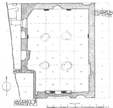
Рис. 2 План развалин мечети в Чуфут-Кале по раскопкам 1928—29 гг.
